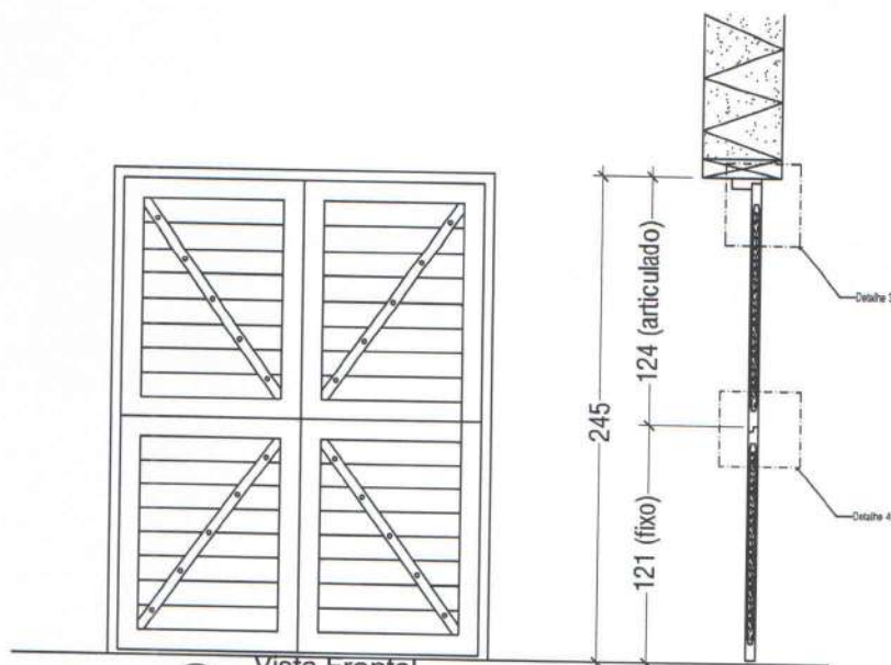
1 Vista Frontal Detalhe Esc. 1:40
