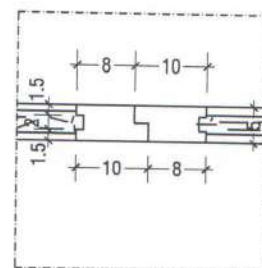
1 Detalhe 2 Detalhe Esc. 1:10
