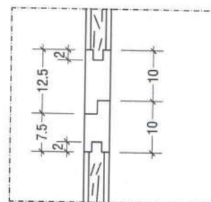
1 Detalhe 4 Detalhe Esc. 1:10
