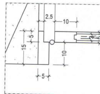
1 Detalhe 1 Detalhe Esc. 1:10
