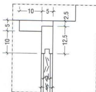
1 Detalhe 3 Detalhe Esc. 1:10
