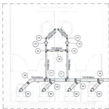
Detalhe 2 Projeto Sanitário Esc. 1/205
