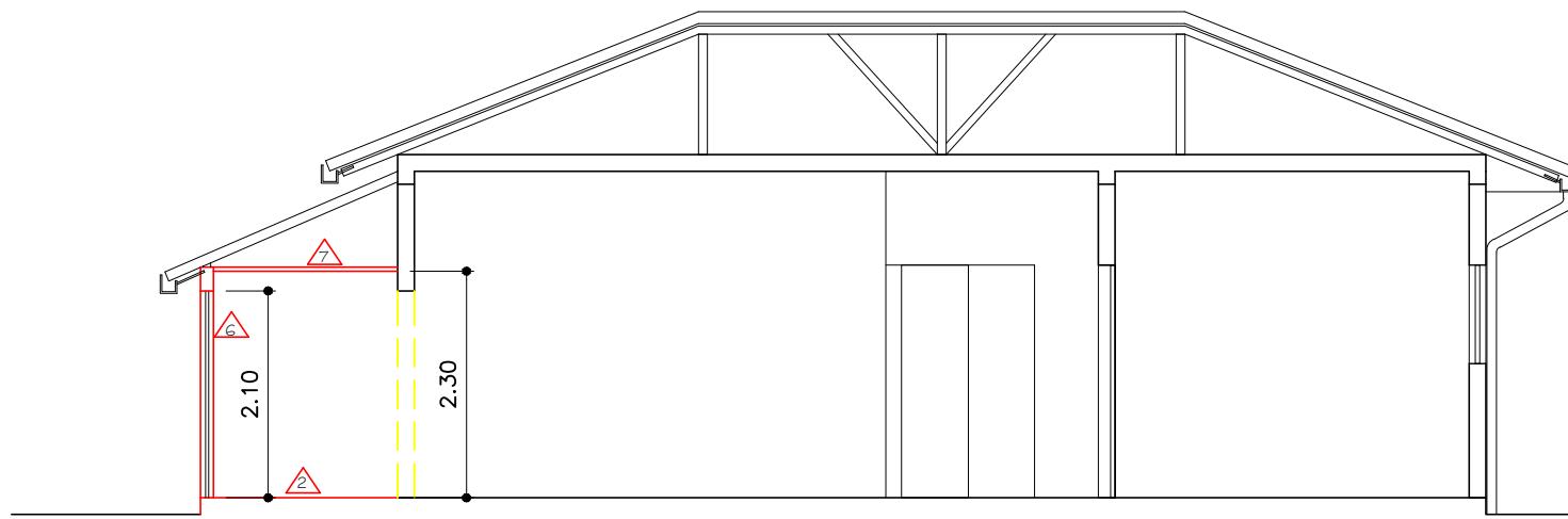
CORTE LONGITUDINAL A - B Escala: 1/75
