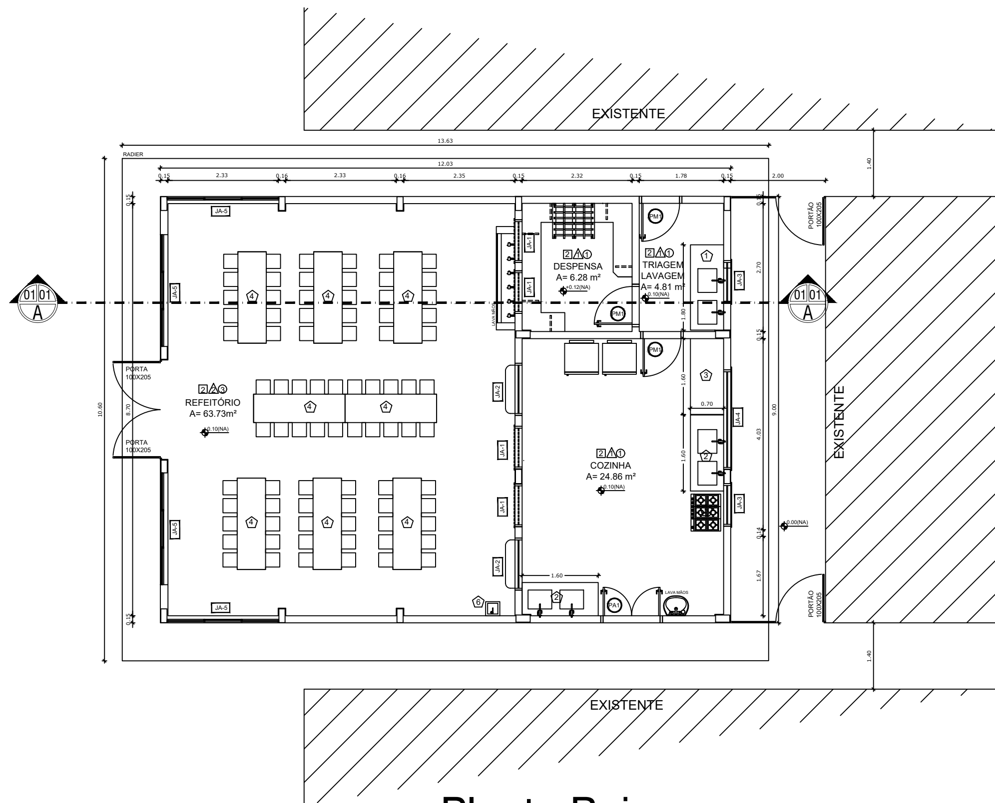
1 Planta Baixa Implantação geral Esc. 1:50
