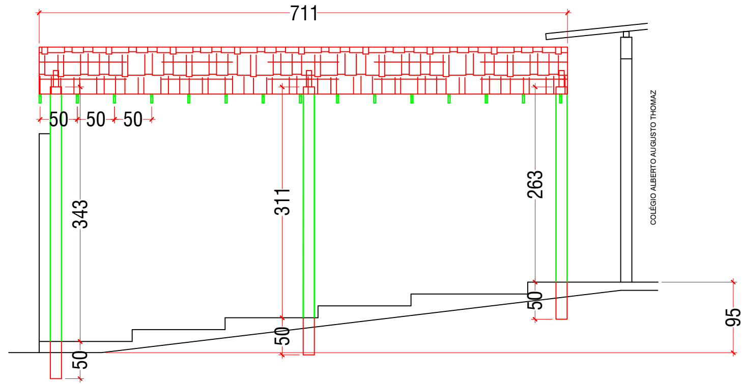
Vista Lateral Esc. - 1:50
