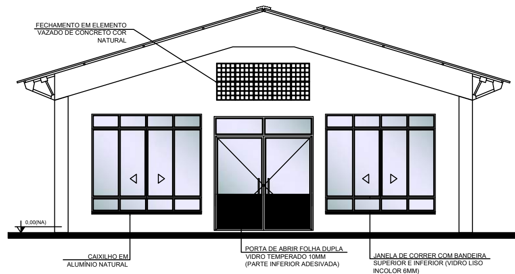
2 Fachada Implantação geral Esc. 1:50
