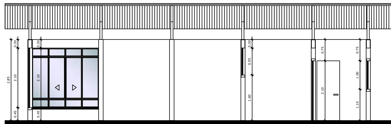
3 Corte A-A Implantação geral Esc. 1:50
