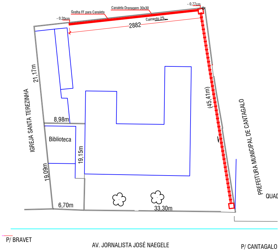
Planta Situação Esc. - 1:500
