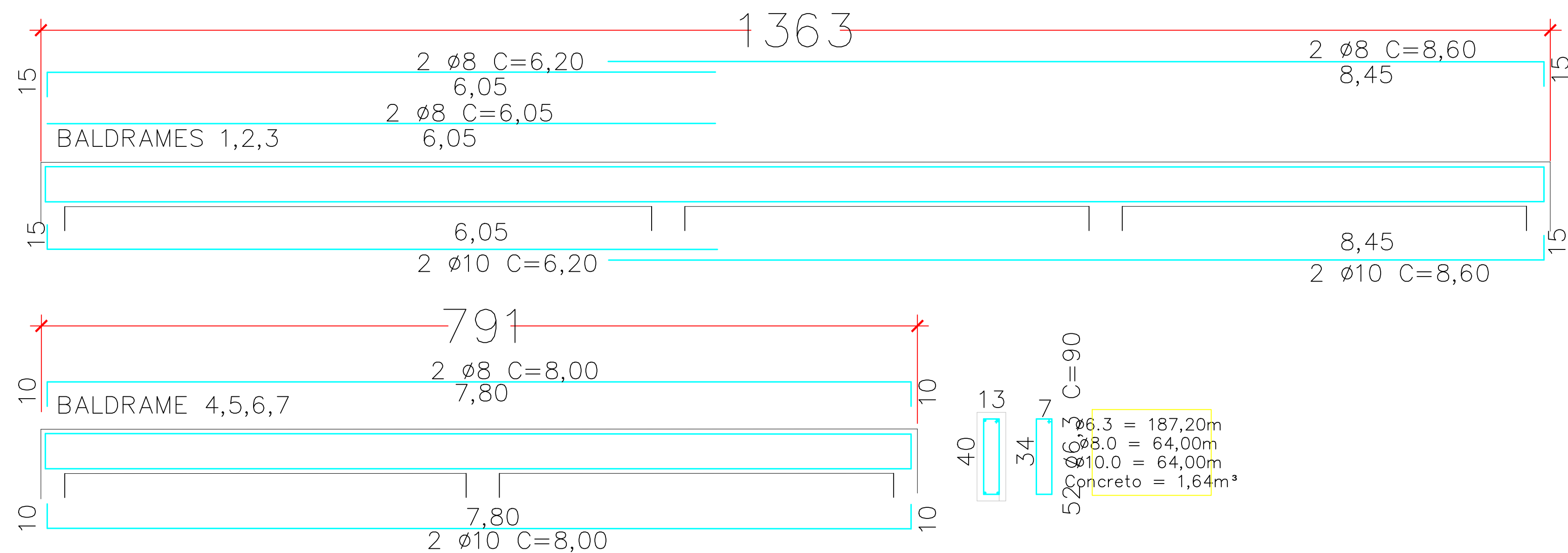
Vigamentos, Sapatas e Tocos de Colunas Esc:1:30
