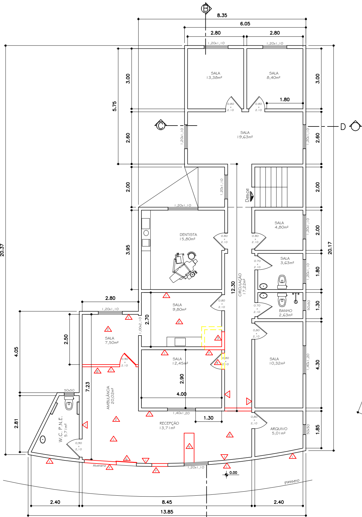
PLANTA BAIXA - TÉRREO Escala: 1/75
