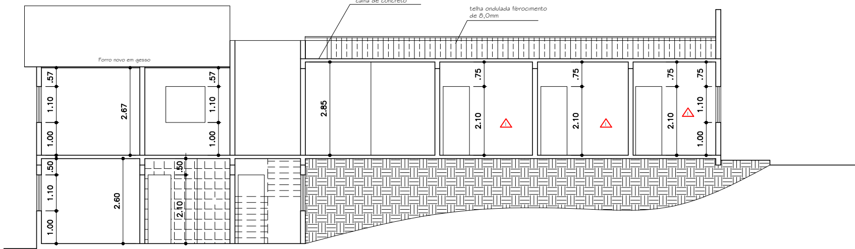
CORTE LONGITUDINAL A - B Escala: 1/75
