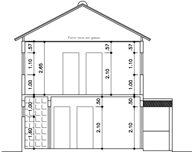
CORTE TRANSVERSAL C - D Escala: 1/75
