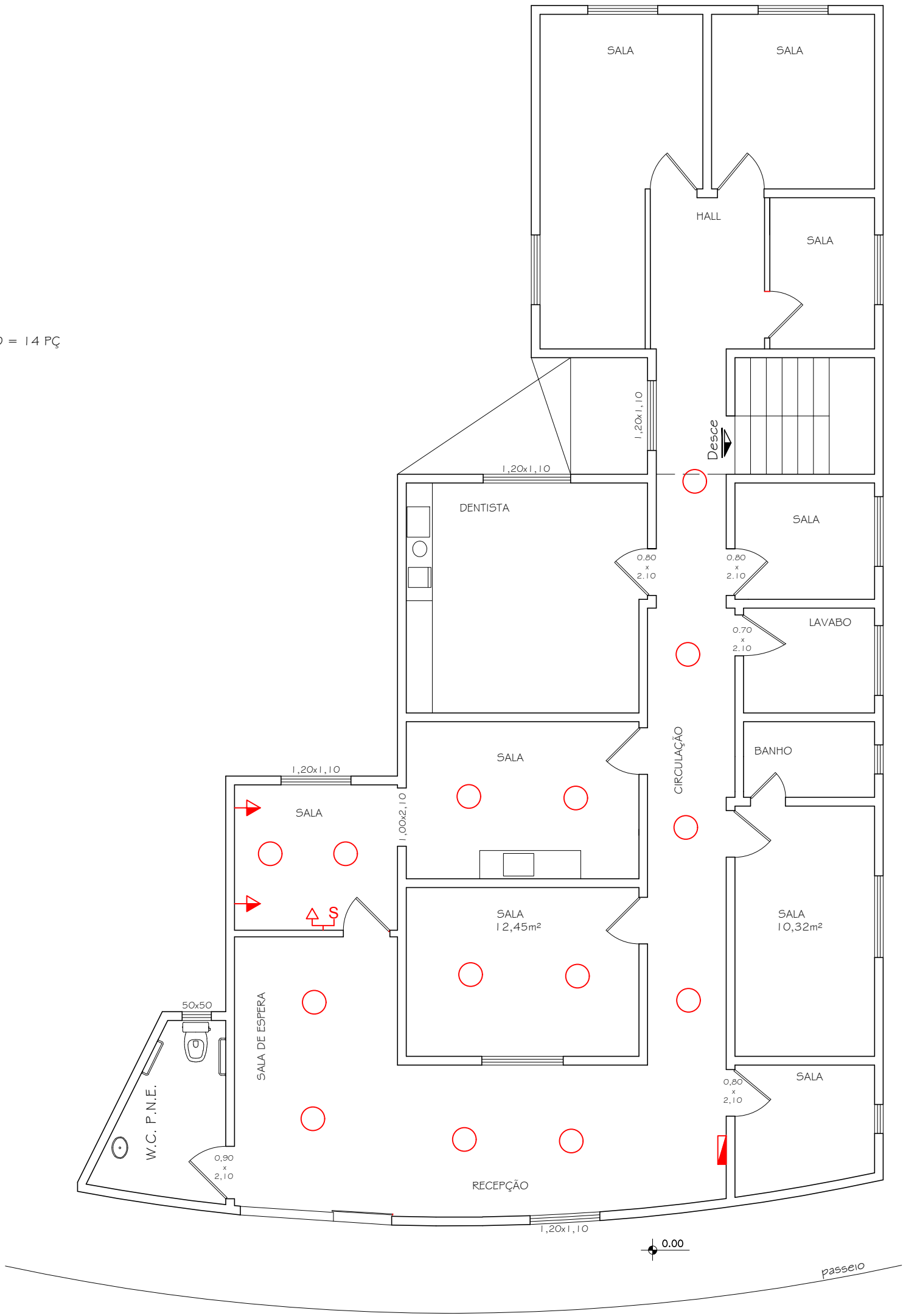
PLANTA BAIXA - TÉRREO Escala: 1/75
