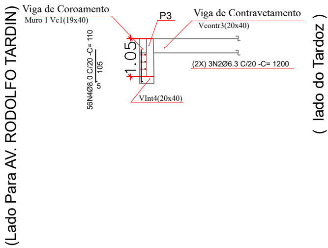
OBS: ÚLTIMO LANCE DA CORTINA (Painéis de 01a 04) MURO 1 ARMAÇÃO DA CORTINA EM BLOCOS ESTRUTURAIS ESCALA 1/100
