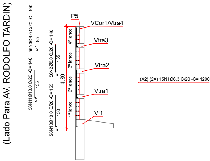
MURO 1 ARMAÇÃO DA CORTINA EM BLOCOS ESTRUTURAIS ESCALA 1/100
