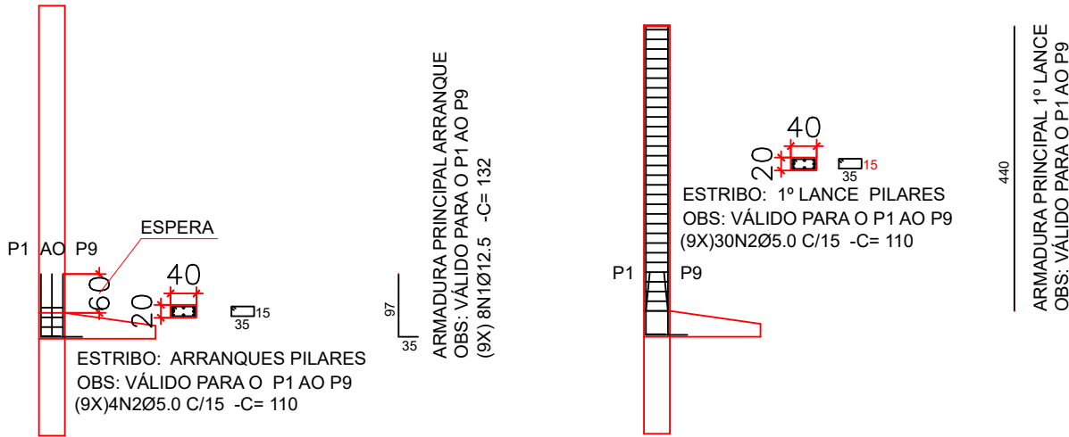
MURO 1 FORMA E ARMAÇÃO PILARES (DO P1 ao P9) ESCALA 1/100
