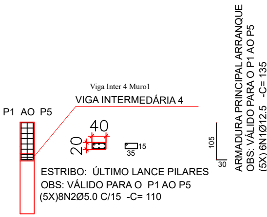
OBS: DETALHAMENTO PELO PILAR MÉDIO MURO 1 FORMA E ARMAÇÃO PILARES (DO P1 ao P5) ESCALA 1/100
