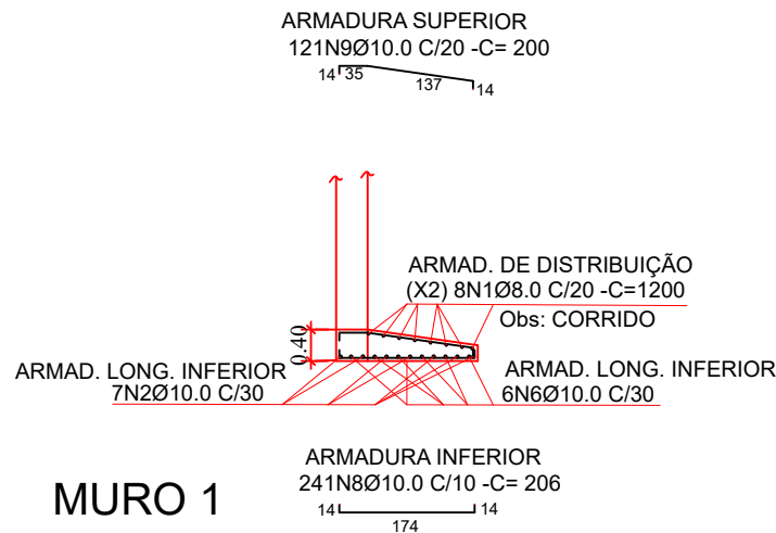
MURO 1 ARMAÇÃO SAPATA SEÇÃO TRANSV. "S1 S1" ESCALA 1/100
