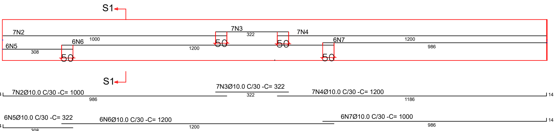
MURO 1 ARMAÇÃO SAPATA CORRIDA S1(1,80X24,00) ESCALA 1/100
