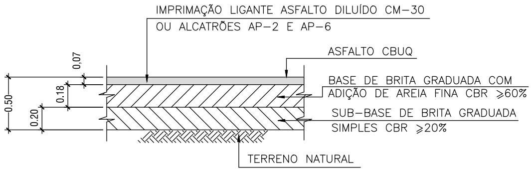
DETALHE 1 PAVIMENTO EM ASFALTO ESC. 1:20
