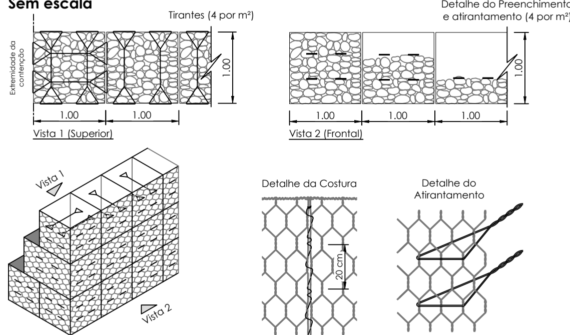
Detalhe 1 : Amarração da Malha e Tirantes Sem escala
