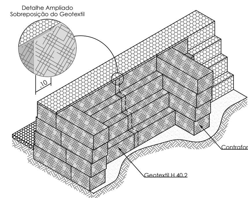
Detalhe 3: Perspectiva esquemática do contraforte Sem Escala
