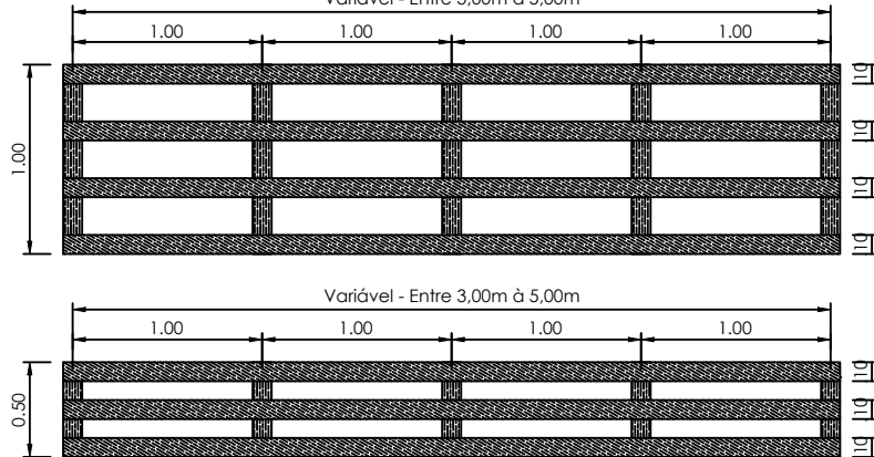
Detalhe dos Gabaritos de Madeira - Altura de 0,50m e 1,00m Sem Escala
