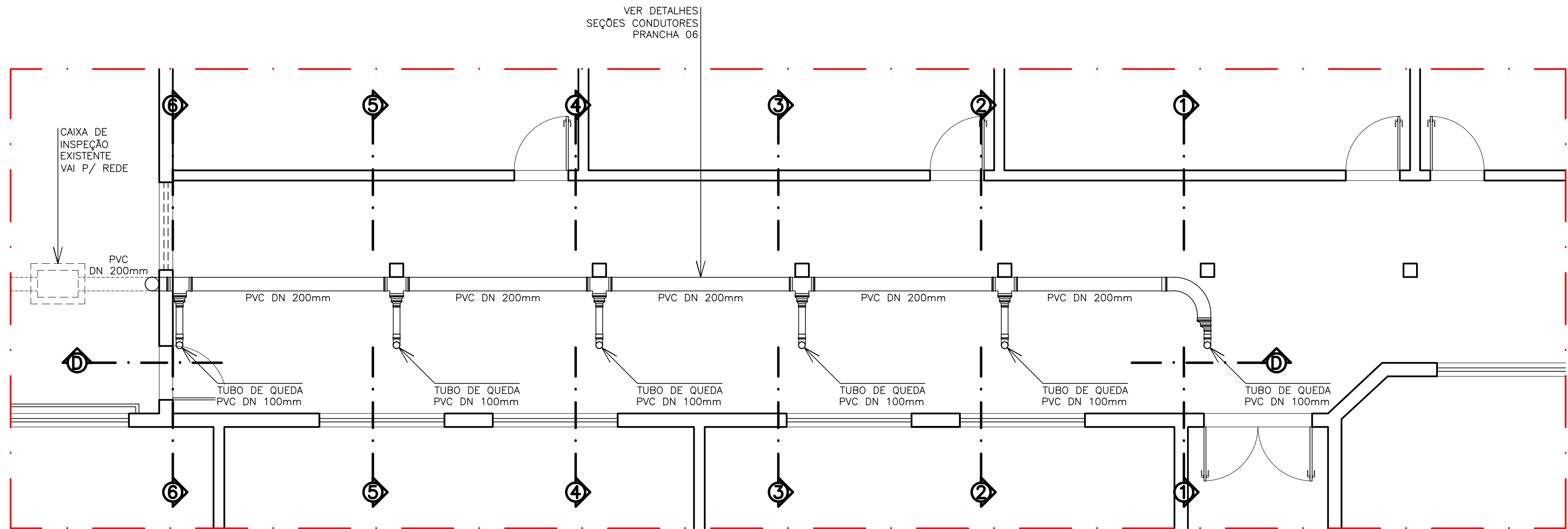
PLANTA BAIXA AMPLIADA LAJE IMPERMEABILIZADA ESC.: 1/50
