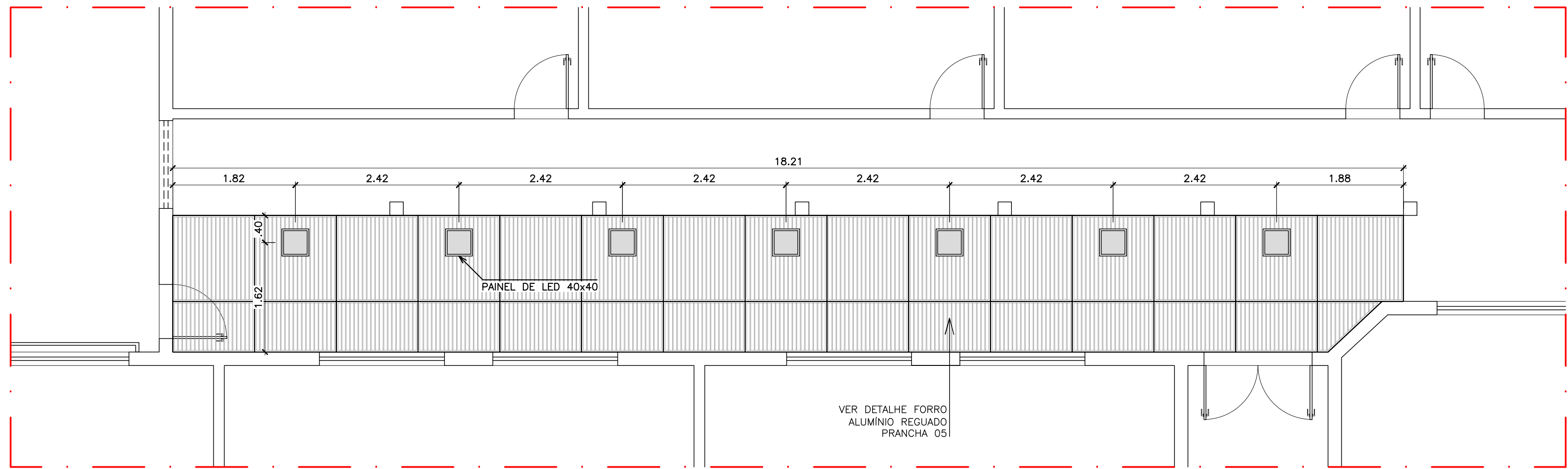
PLANTA BAIXA AMPLIADA FORRO TETO / ILUMINAÇÃO ESC.: 1/50
