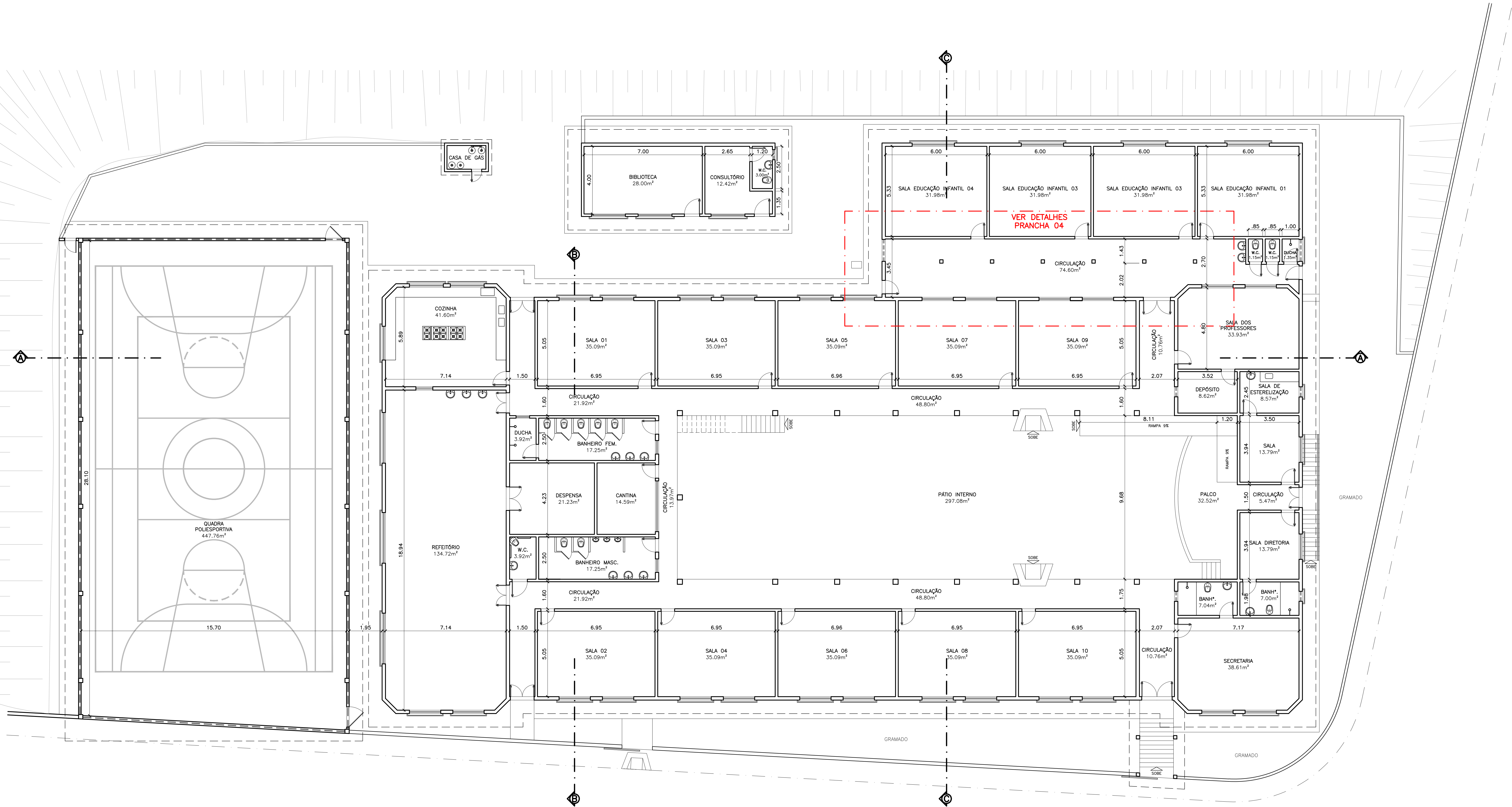
PLANTA BAIXA PAVT* TÉRREO ESC.: 1/100
