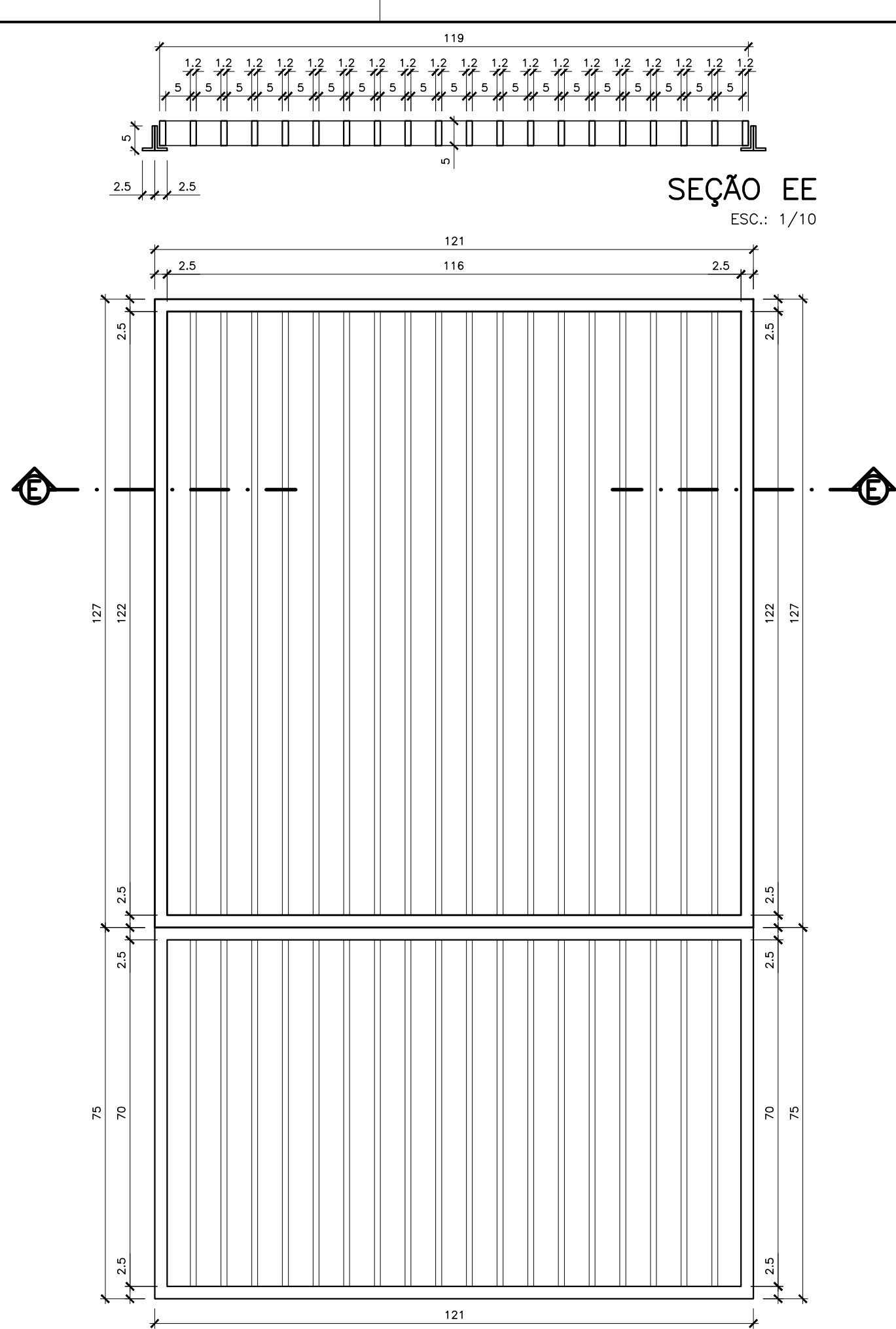
DETALHE FORRO ALUMÍNIO REGUADO ESC.: 1/10 OBS.: Colas em cm.
