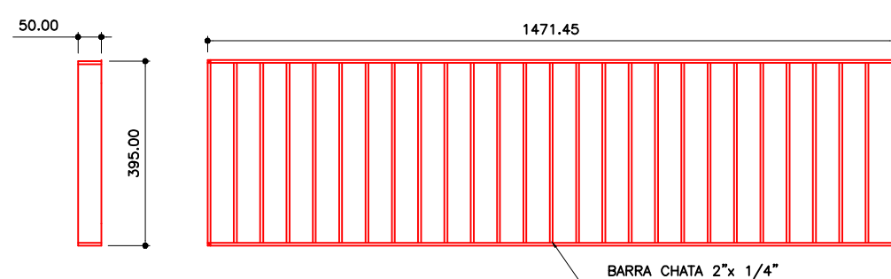
GRADE DA CANALETA Escala.: 1:10
