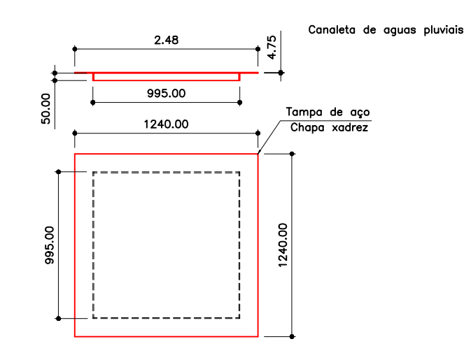
PLANTA - TAMPA DA CX DE PASSAGEM - CHORUME Escala.: 1:25 - (Medidas em Milímetros)
