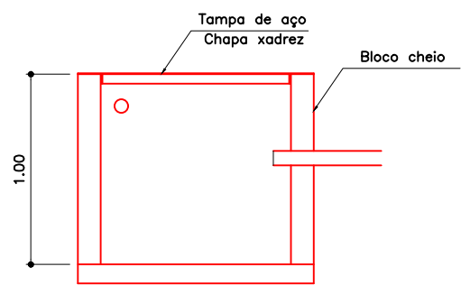
PLANTA - TAMPA DA CX DE PASSAGEM - CHORUME Escala.: 1:25 - (Medidas em Milímetros)
