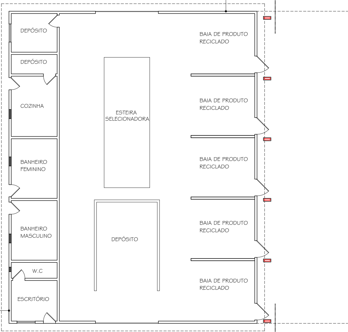
PLANTA BAIXA (USINA) Escala.: 1:100
