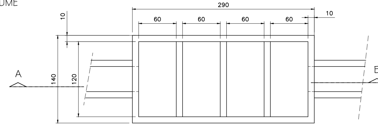
PLANTA - MEDIDAS EM CENTÍMETROS Escala.: 1:25
