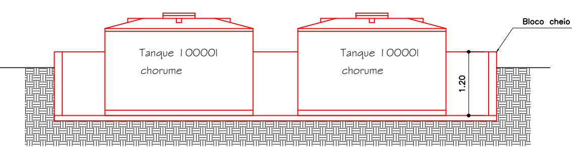
CORTE A-B (DIQUE) Escala.: 1:50
