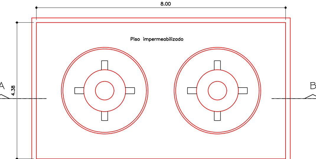
PLANTA - DIQUE E TANQUES DE 10000l Escala.: 1:50
