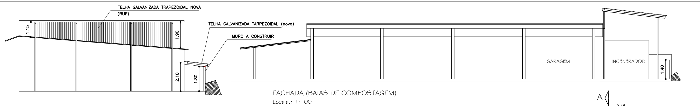
CORTE A-B (INCINERADOR) Escala.: 1:100
