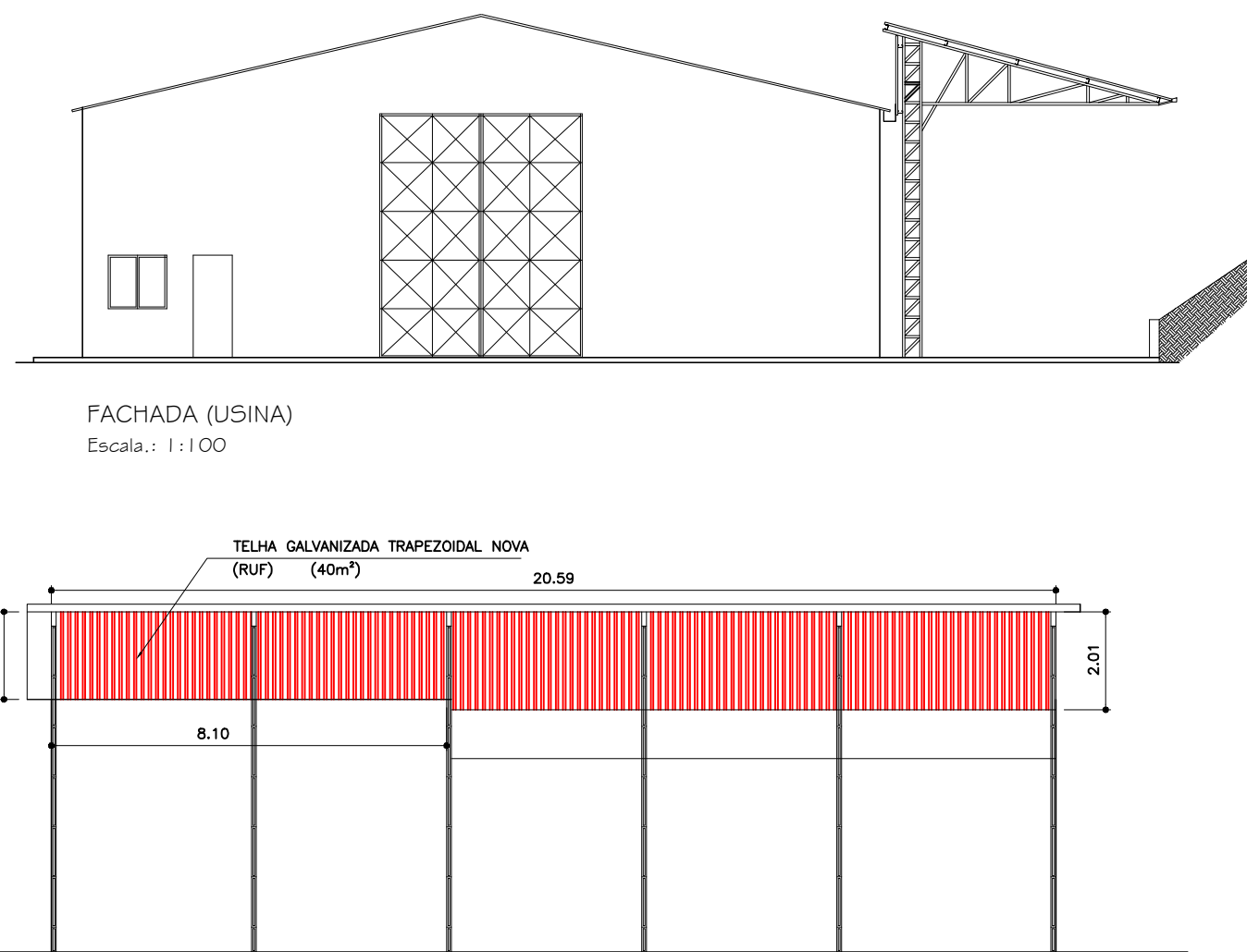
CORTE A-B (USINA) Escala.: 1:100
