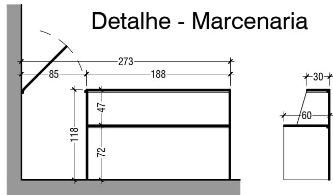
MARCENARIA EM COMPENSADO 15mm ACABADO COM MASSA E PINTURA
