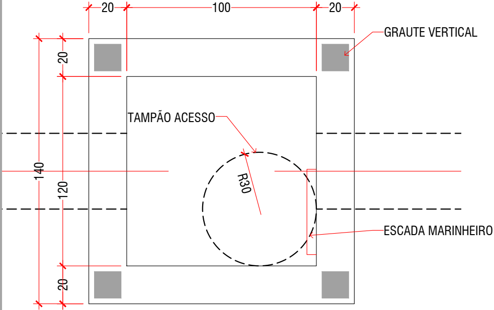
Det. Poço de Visita Esc: 1:20
