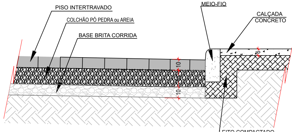
2 Detalhamento Esc. 1:20
