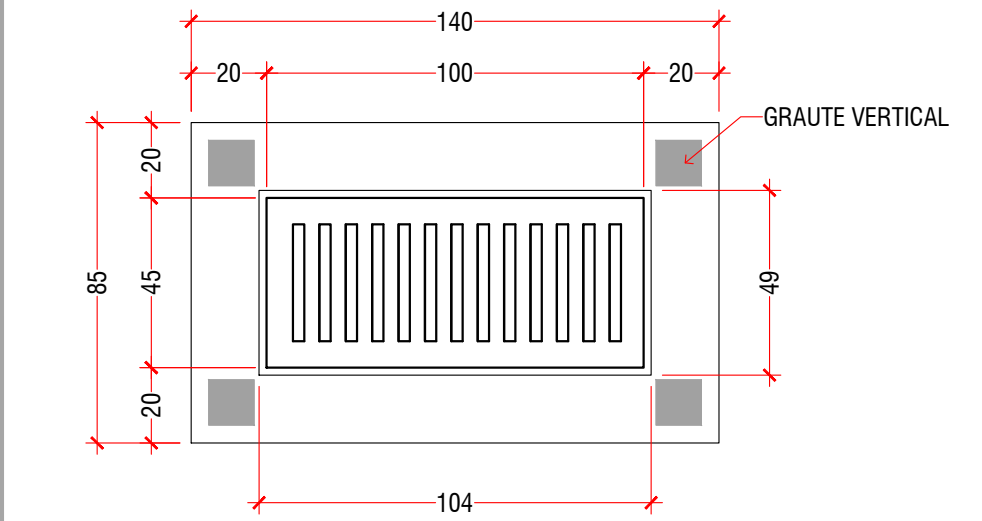
Det. Boca de Lobo Esc: 1:20
