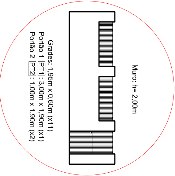
DETALHAMENTO DO MURO ESC.: 1:100
