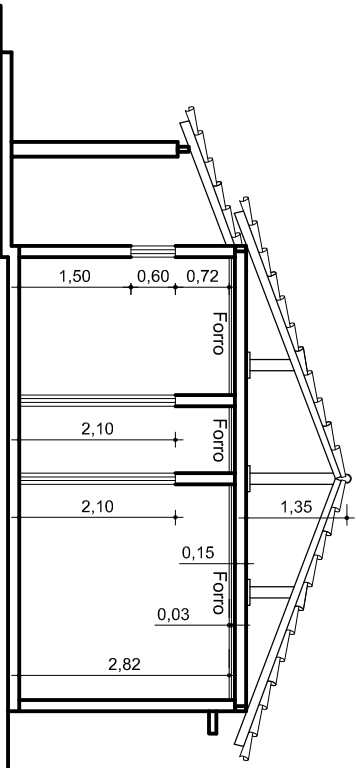
CORTE A-A ESC.: 1:100
