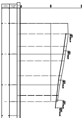
R. JOÃO GERK PERFIL DAS REDES
