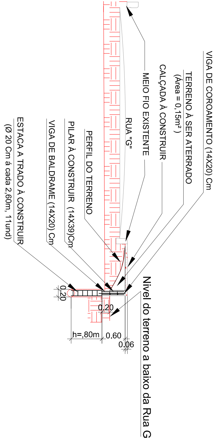
SEÇÃO: "S2 S2"
