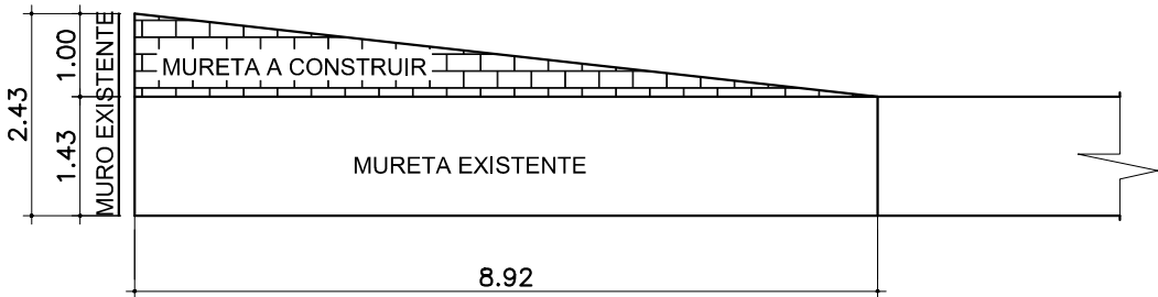
PROLONGAMENTO DE MURETA ARMADA
