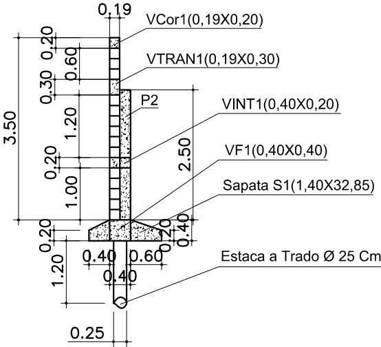
SEÇÃO S1S1 ESCALA 1/100
