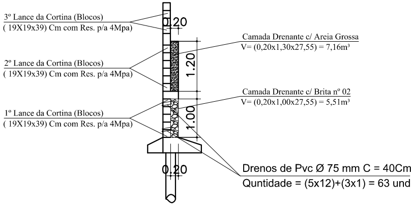
SEÇÃO S3S3 ESCALA 1/100
