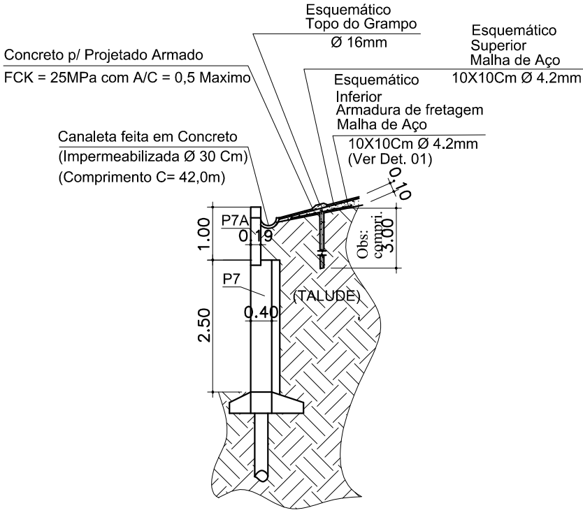
SEÇÃO S2S2 ESCALA 1/100
