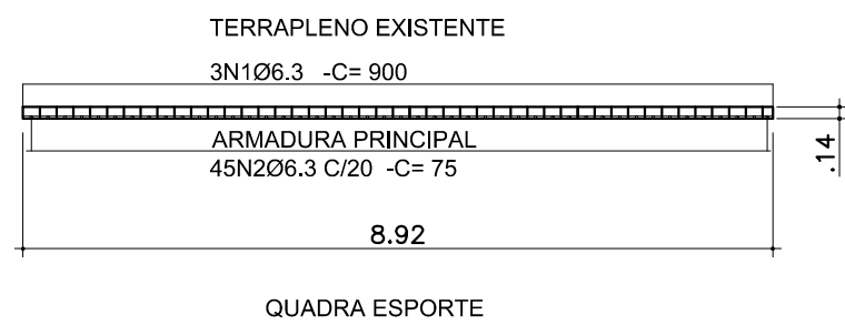
ARMAÇÃO: PROLONGAMENTO DA MURETA
