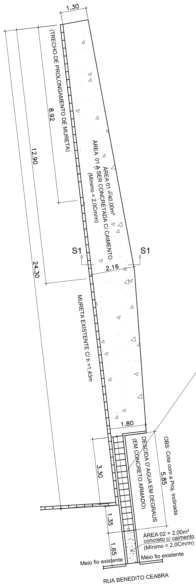
CIMENTADO ARMADO E DESCIDA D'AGUA EM DEGRAUS
