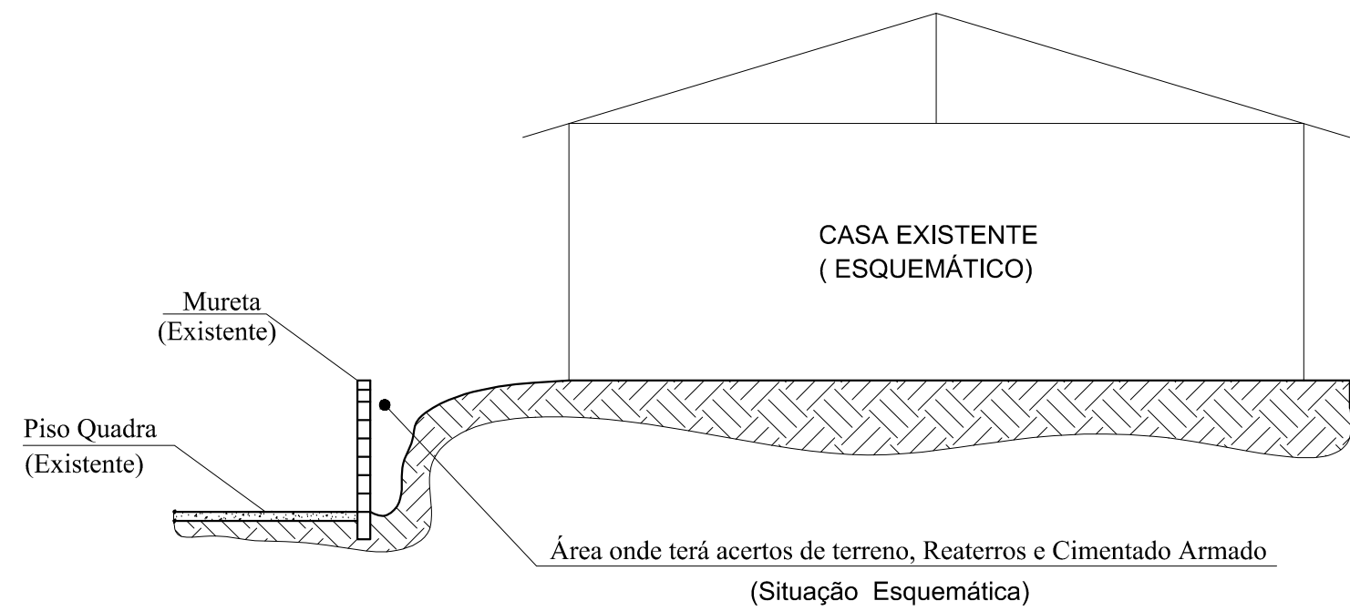
SEÇÃO S1S1 DA ÁREA 01 DO CIMENTADO ARMADO
