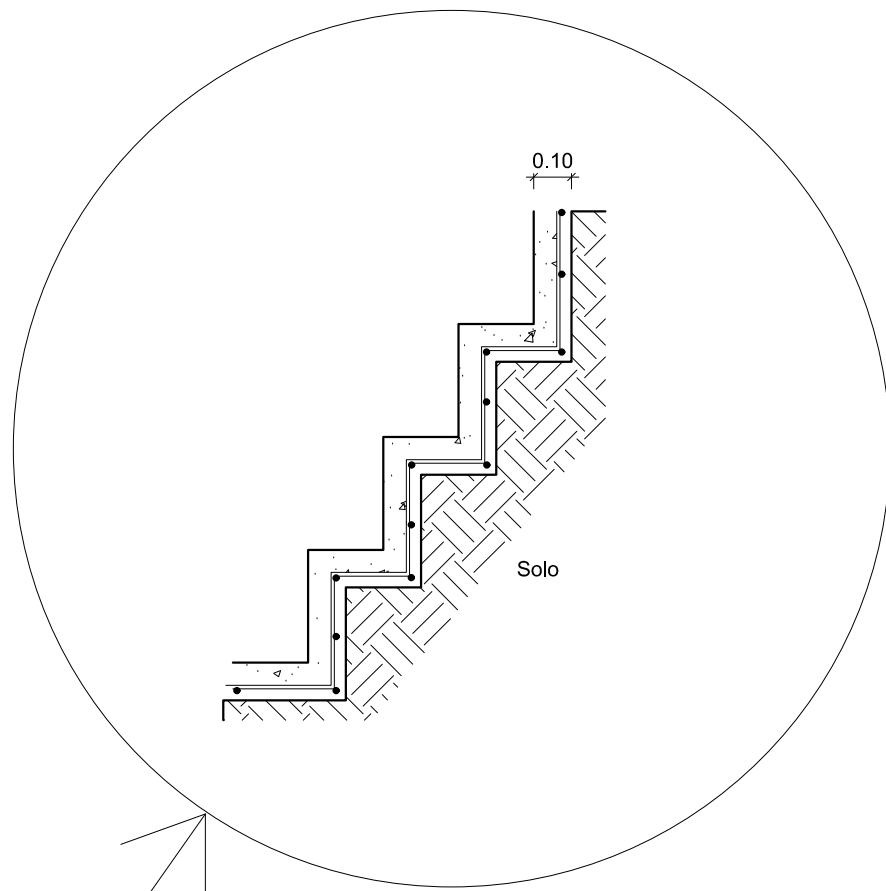
DETALHE DA DESCIDA D'ÁGUA EM DEGRAUS
